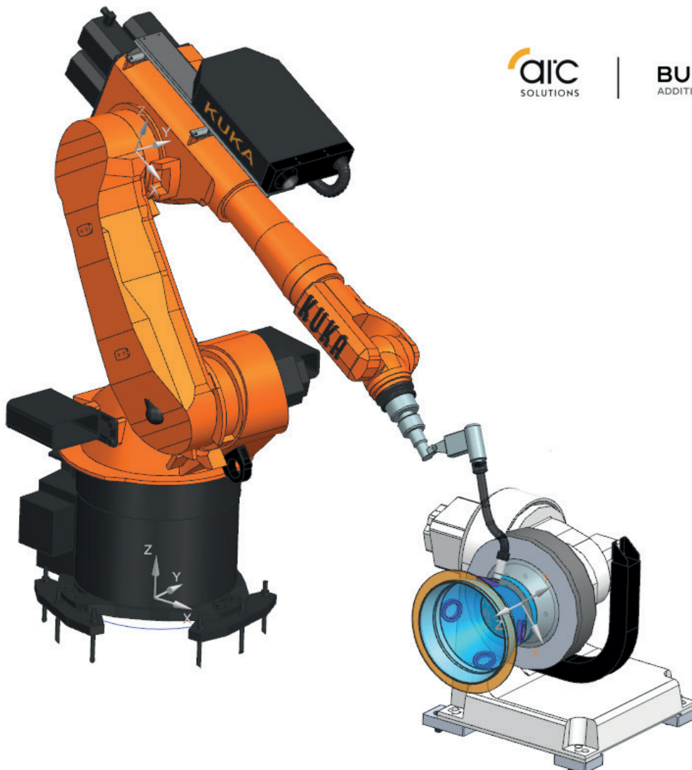
mit Roboter additiv gefertigtes Bauteil
